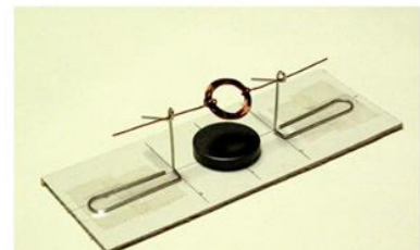
組立てられたモーター
